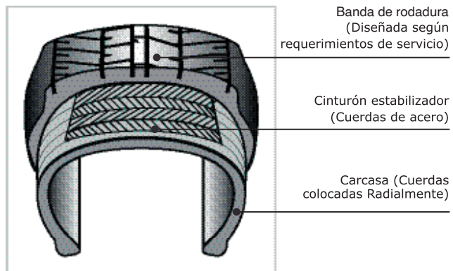
Construcción Radial
