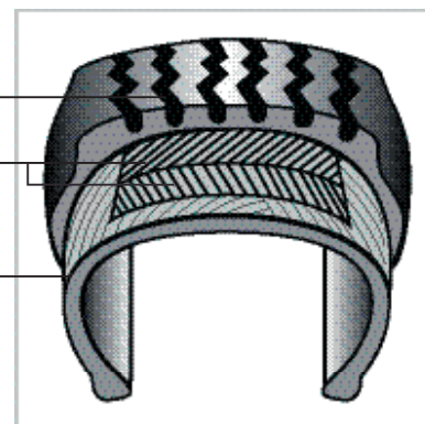
Construcción Convencional
